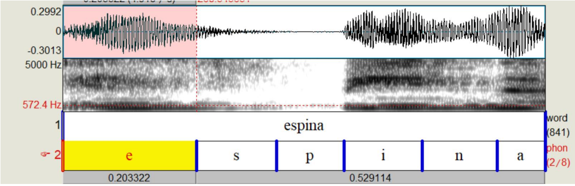
Imagen 5: oscilograma, espectrograma y etiquetado del informante 06_M_A2_PE en la producción de [ɛ] en “ espina ”
