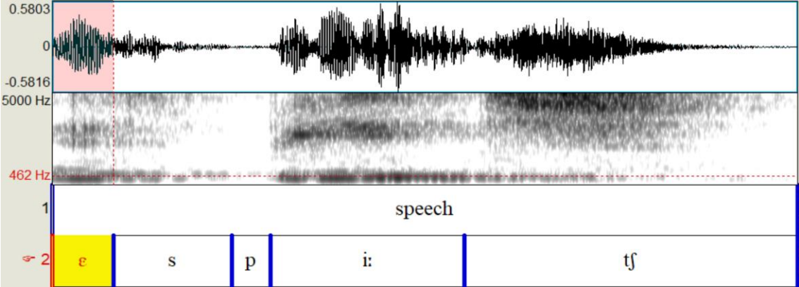
Imagen 4: Oscilograma, espectrograma y etiquetado del informante 06_M_A2_PI en la producción de VE en “ speech ”
